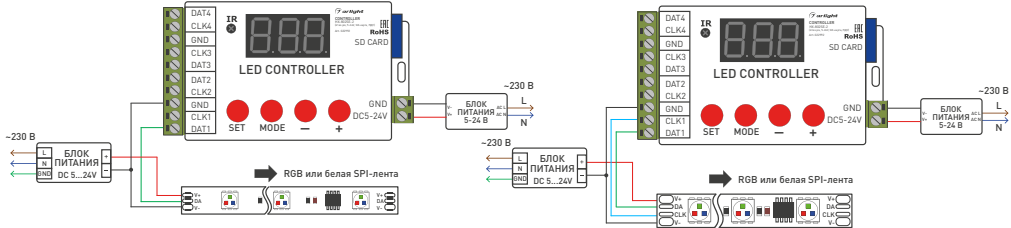
Рис. 1. Подключение SPI-лент к контроллеру
