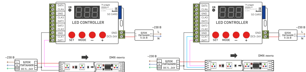
Рис. 2. Подключение DMX-лент к контроллеру
