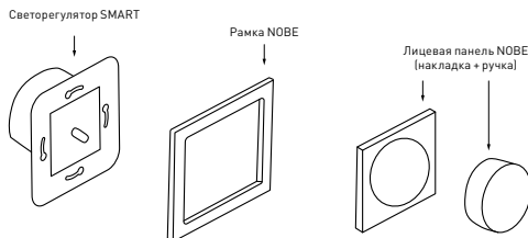
Рис. 5. Монтаж светорегулятора
