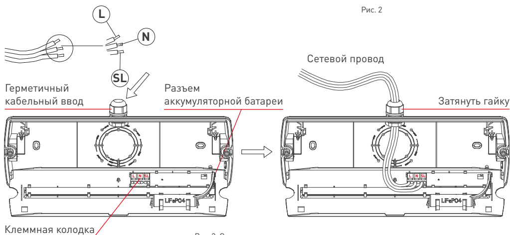
Рис. 3. Стандартная схема подключения
