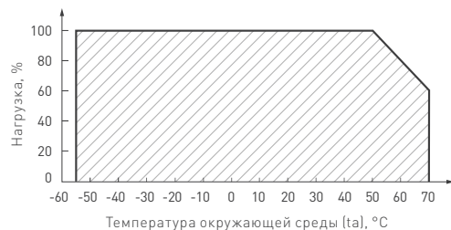
Рис. 2. Максимальная допустимая нагрузка, % от мощности источника
