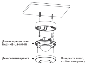
Рис. 4. Схема монтажа
