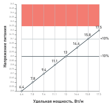
График 1. Зависимость удельной мощности от напряжения питания
