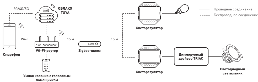
Рис. 2. Структурная схема построения системы
