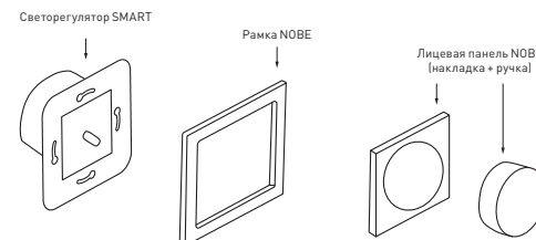
Рис. 5. Монтаж светорегулятора
