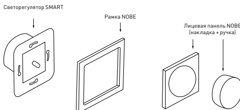
Рис. 5. Монтаж светорегулятора
