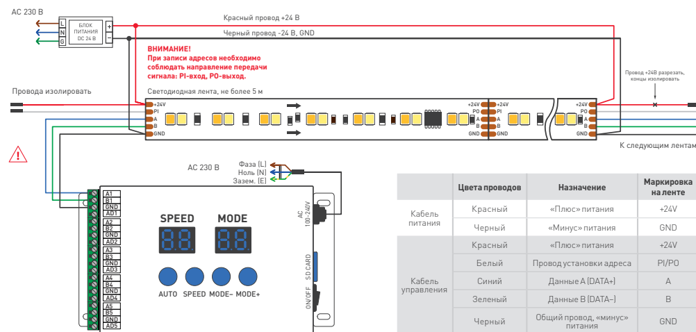
Схема 1. Подключение ленты с использованием контроллера с несколькими портами и с функцией редактирования адресов
